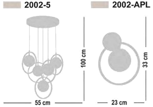
2002-APL E14 / 1 x 40W Max.
