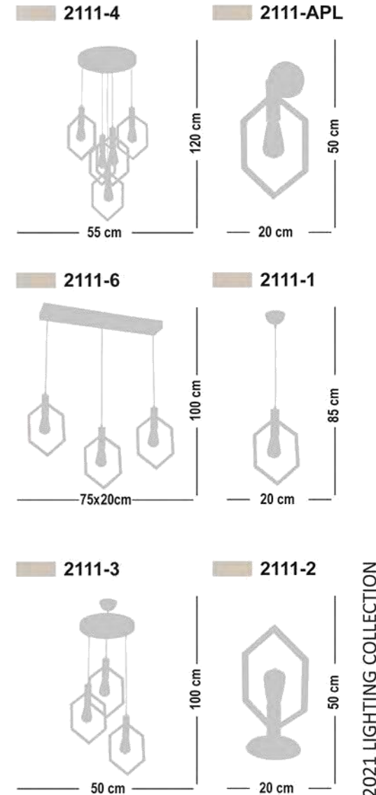
2111-APL E27 / 1 x 60W Max.
